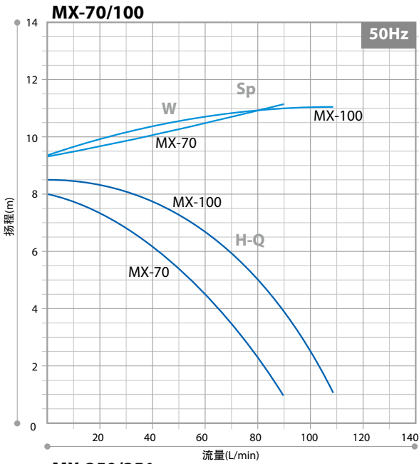
性能曲线 (以下数据仅供参考，请向易威奇索要正规性能曲线。)
